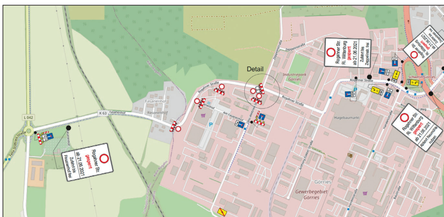
Verkehrszeichenplan der Baumaßnahme Rogahner Straße
