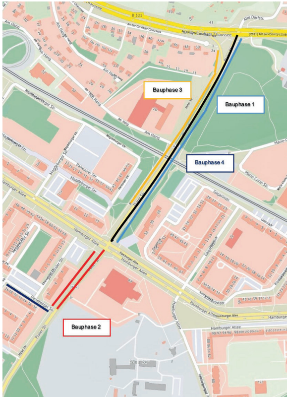
Lageplan der verschiedenen Bauphasen der Instandsetzung in der Plater Straße
